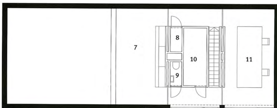
PLANTA PRIMERA
