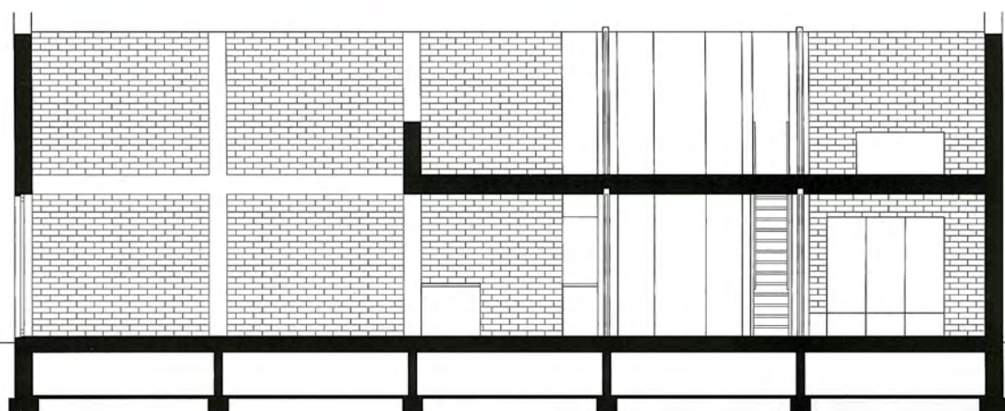
SECCIÓN LONGITUDINAL
