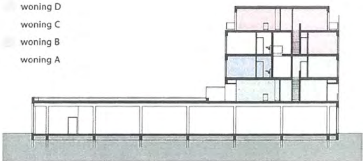
DOORSNEDEAA' SINT-GUMMARUSSTRAAT
